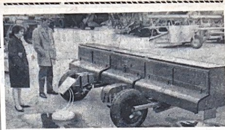
МОСКВА. Конструкторы завода «Красная Звезда» Приднепровского совнархоза представили на Выставку достижений народного хозяйства СССР тракторную селву «РТТ-42». Новая машина предназначена для расчистки на поверхности почвы минеральных удобрений, их смесей и известки, а также для подкормки зерновых культур.
